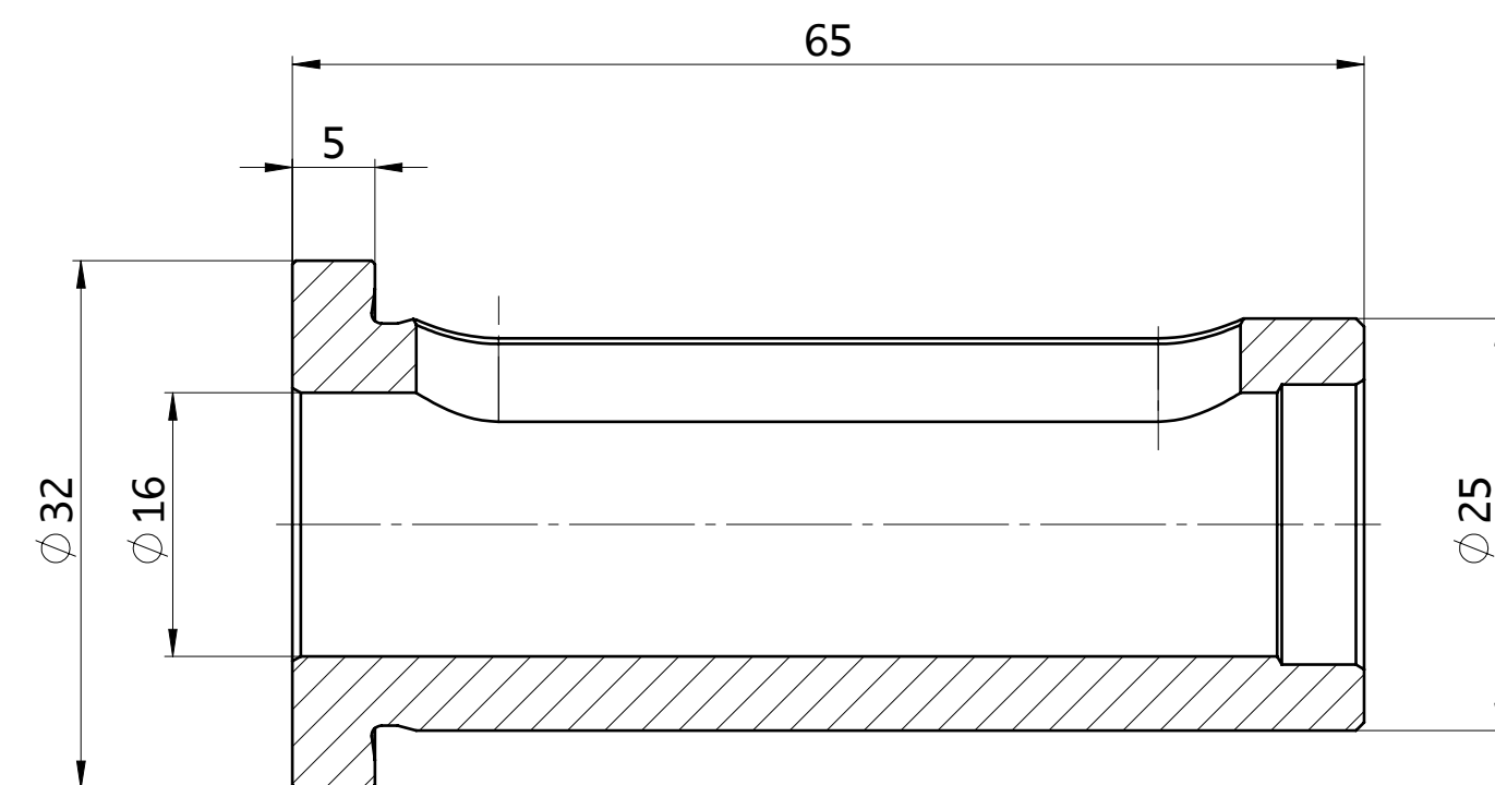
SEZIONE A-A
